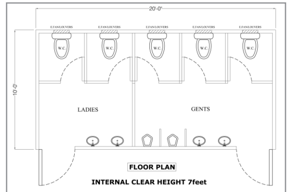
Portable Toilet
